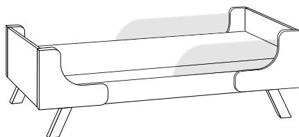
Bett niedrig oder Gitterbett umgebaut und mit Verlängerungsset L x B x H: 1650 x 750 x 520 mm, Matratze 1600 x 700 mm
